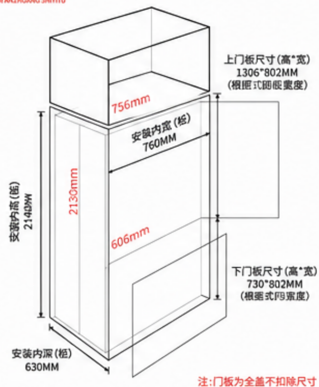
全嵌款及安装示意图 AIOXKUAN JI ANCHUANG SHIYITU
